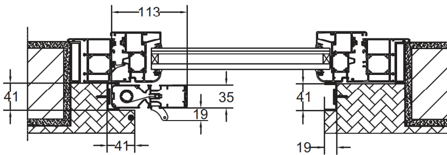
CUFFIA SUPERIORE UNI SENZA UN' ALETTA APPLICAZIONE INCASSO DA 40 mm COMPLANARE AL SERRAMENTO
