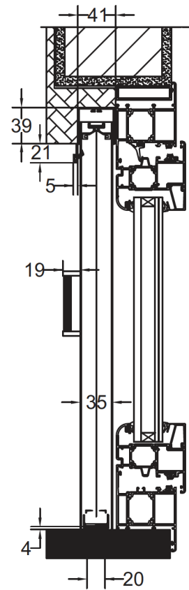
CUFFIA SUPERIORE UNI SENZA UN' ALETTA APPLICAZIONE INCASSO DA 40 mm COMPLANARE AL SERRAMENTO
