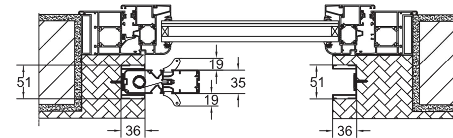
CUFFIA SUPERIORE UNI APPLICAZIONE INCASSO DA 50 mm STANDARD
