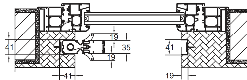
CUFFIA SUPERIORE UNI APPLICAZIONE INCASSO DA 40 mm STANDARD
